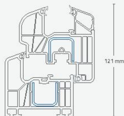
Dorazové těsnění (AD) Obr.: 1:2,5
