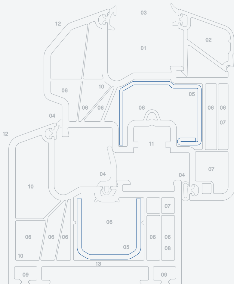
Prestige aktuální varianta I 76.6 C4 Těsnění uprostřed (MD)
