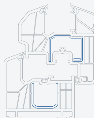
Prestige aktuální varianta I 76.6 C4 Těsnění na dorazu (AD)
