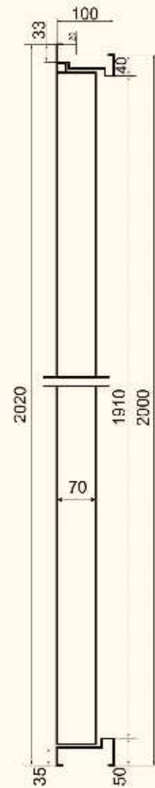
Zvislý rez
