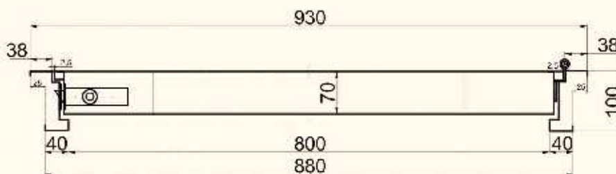
Vodorovný rez
