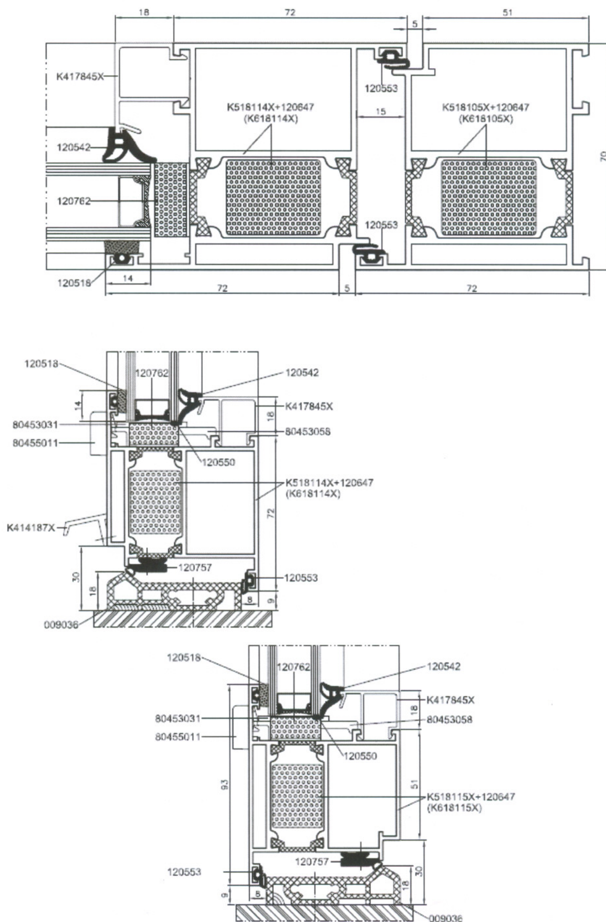
Obrázek 1 – Řez dveřmi
